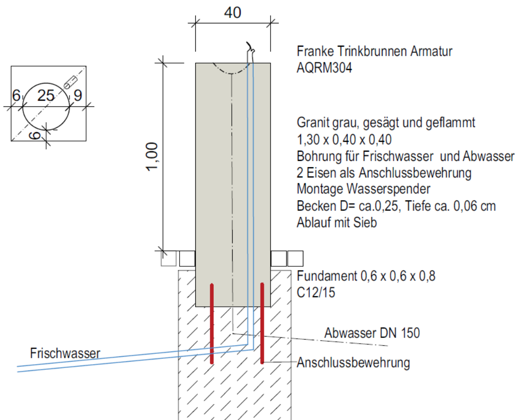
Detail Trinkbrunnen M. 1:20
