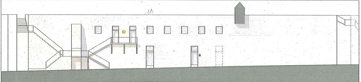
Ansicht Süd
