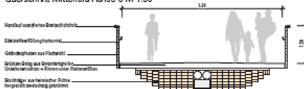
Querschnitt Mittelfeld Achse 3 M 1:50
