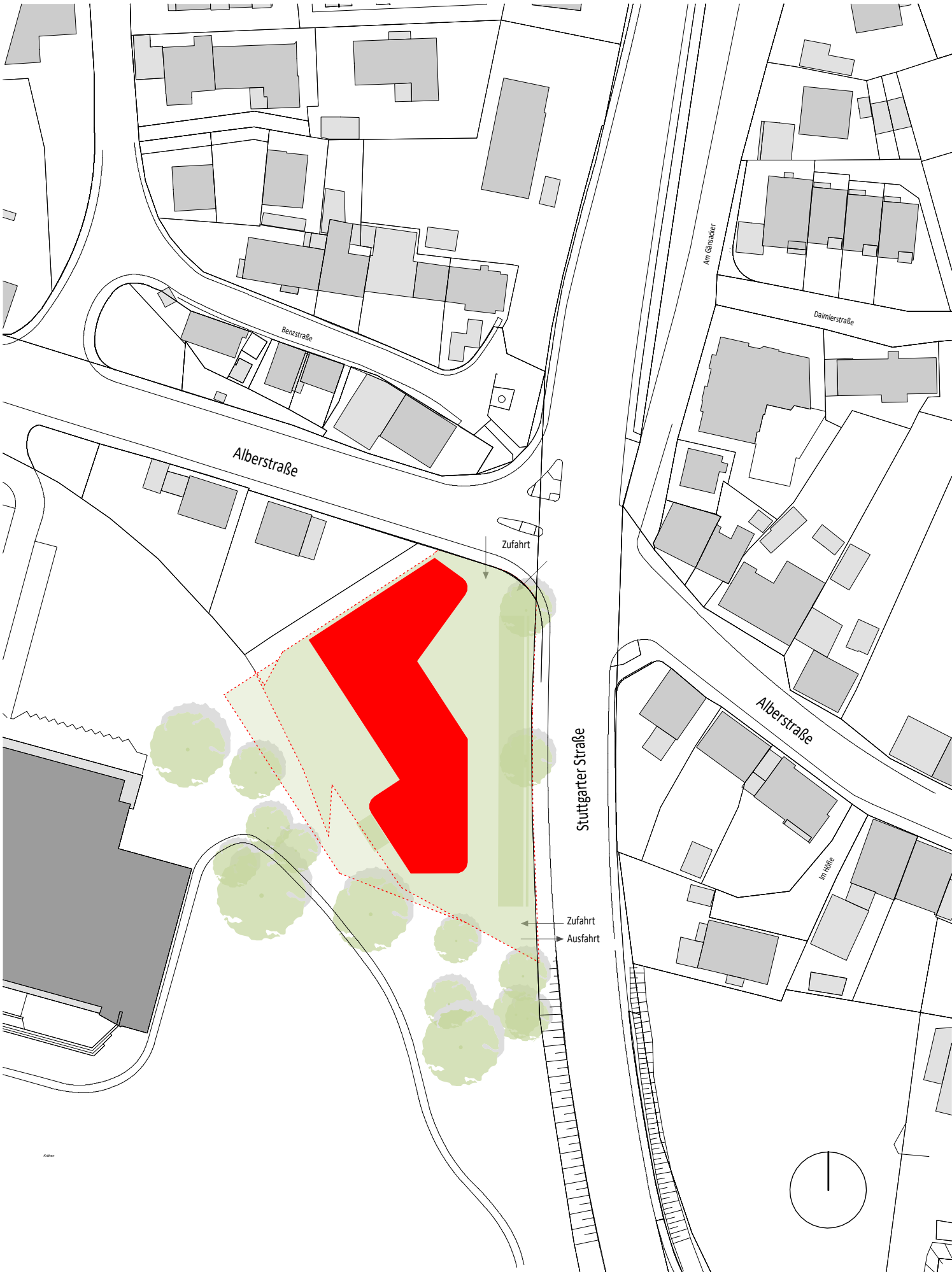
Neubau Feuerwehrhaus Lustnau, Entwurf Lageplan
