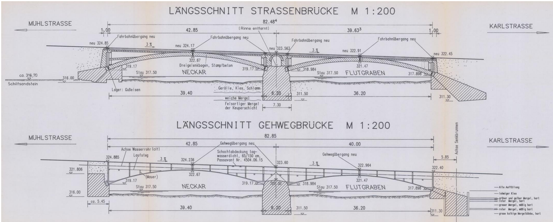
Übersichtsplan: Längsschnitte Eberhardsbrücke
