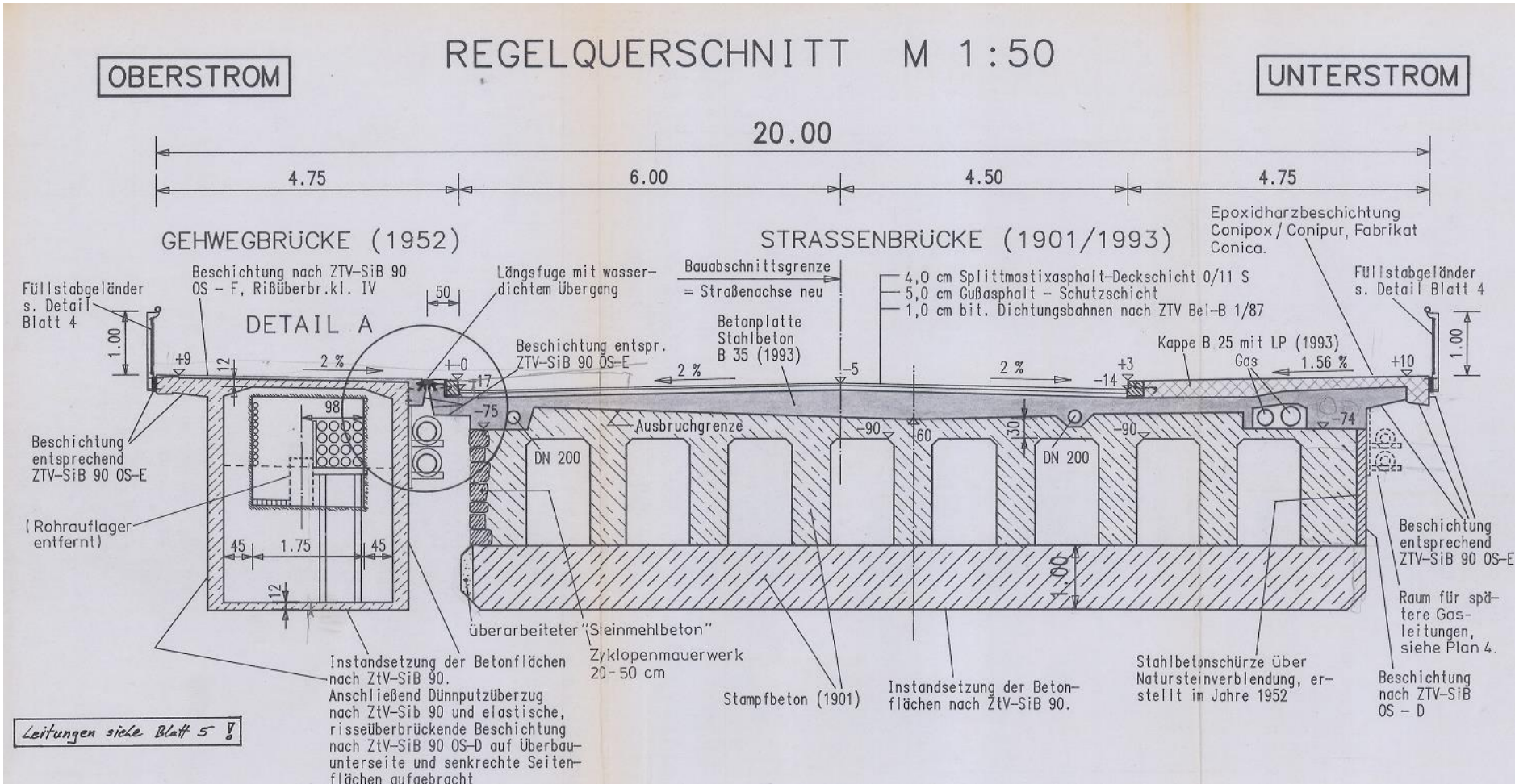
Übersichtsplan: Querschnitt Eberhardsbrücke
