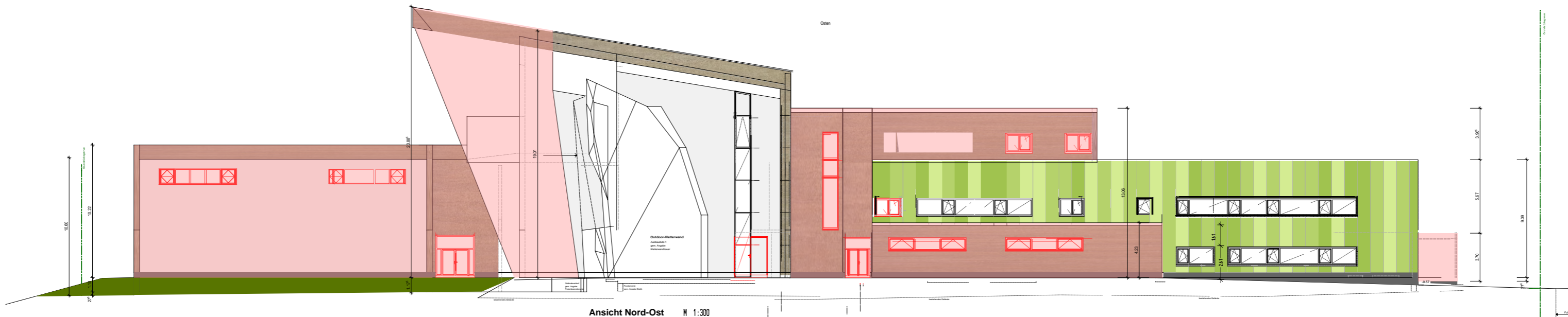
Ansicht Nord-Ost M 1:300
