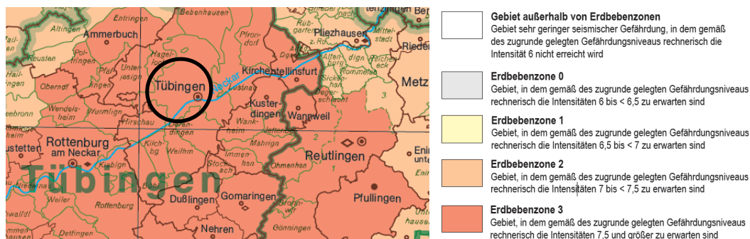
Abb. 3: Karte der Erdbebenzonen und geologischen Untergrundklassen für Baden-Württemberg 1:350.000 (Innenministerium Baden-Württemberg, 2005)
