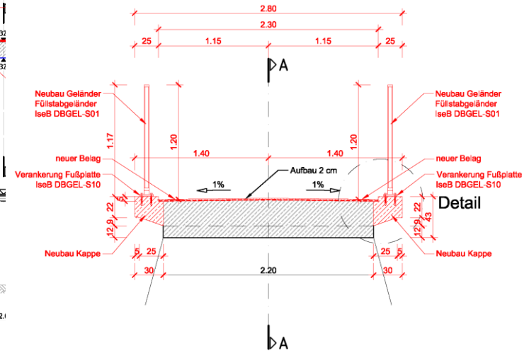
Querschnitt in Brückenmitte Fußgängerbrücke M 1:25
